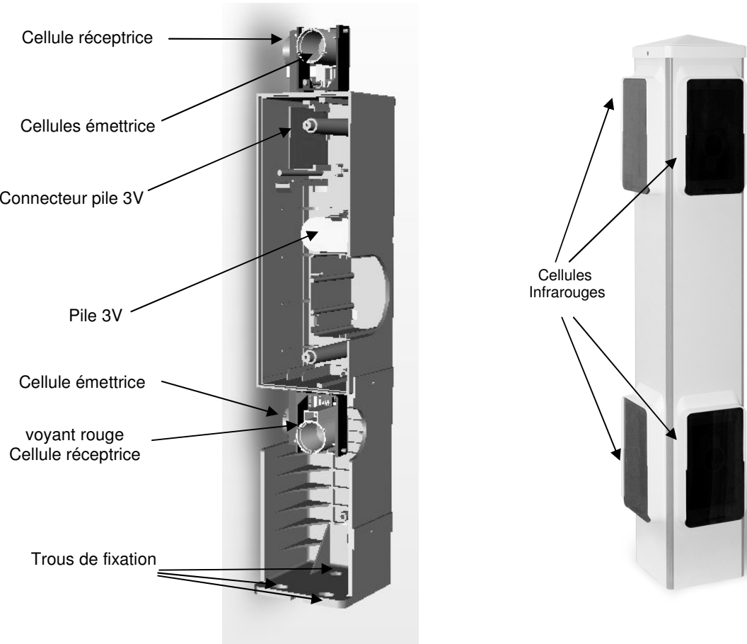
Figure 4 : borne esclave
